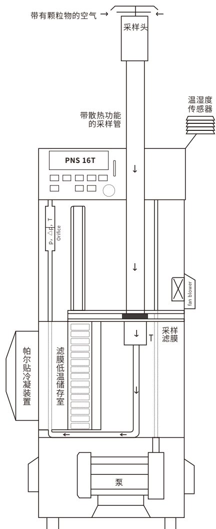
产品结构图
