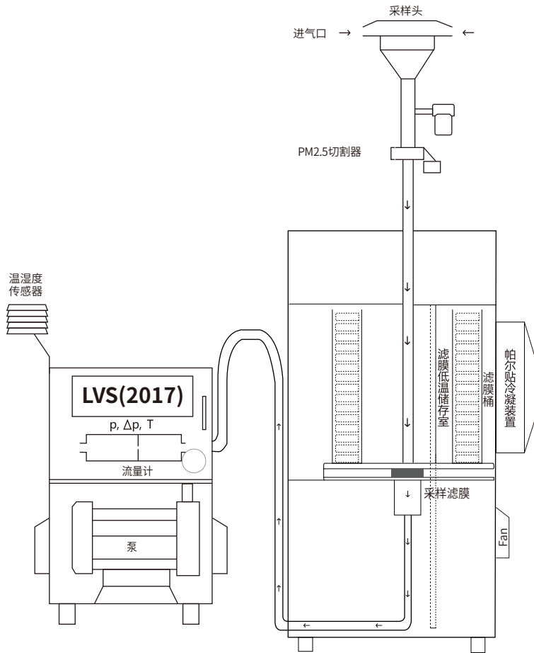
产品结构图
