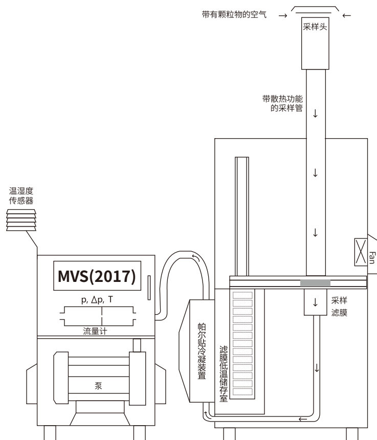
产品结构图
