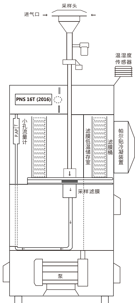
产品结构图
