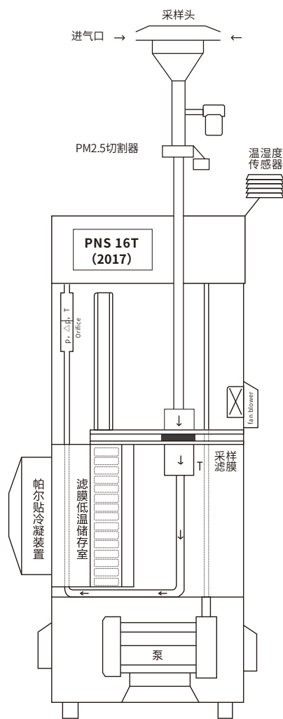
产品结构图
